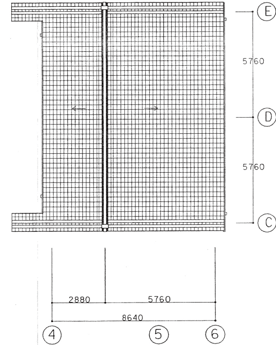
屋根伏図
